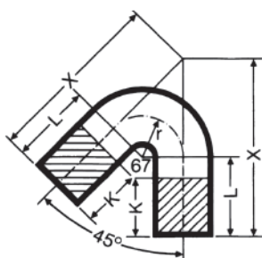
Отвод для обводных трубопроводов 135° PAM-GLOBAL® S
