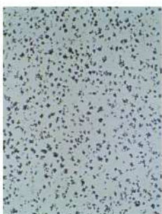
СЭМ (сканирующий электронный микроскоп) - фото: Образование графита розеточной формы труб PAM-GLOBAL®
